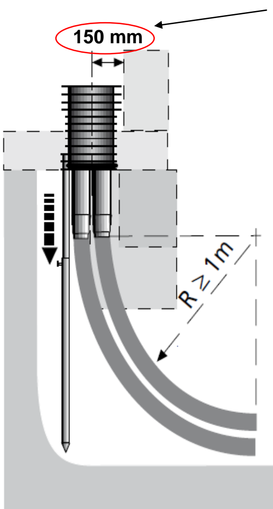
Reiheninstallation 4-fach
